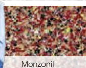
Monzonit
